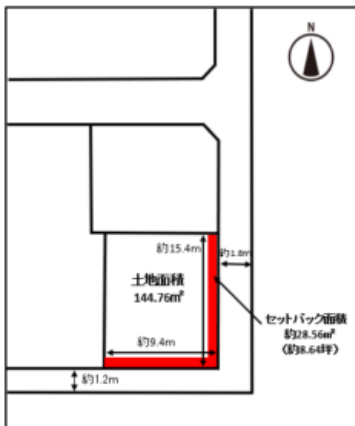
「敷地概略図」
