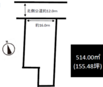
【地形図】
